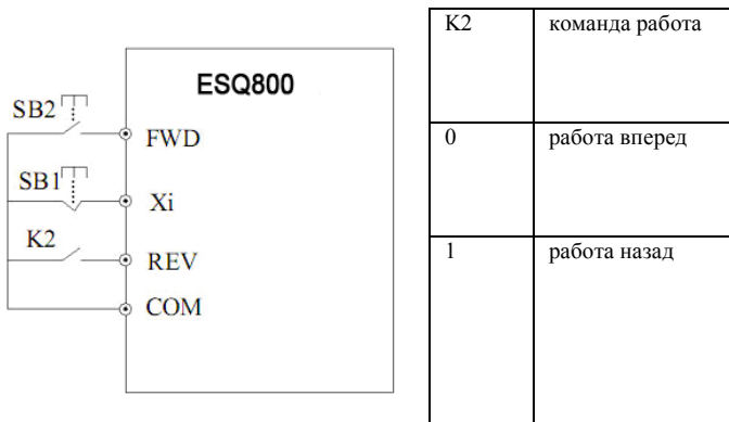
Рис. 6-30 2-проводной режим работы 3
