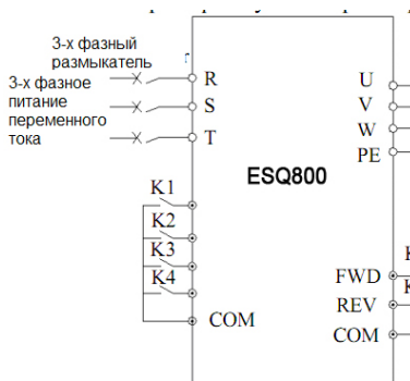
Рис. 6-25 работа на многоступенной скорости
