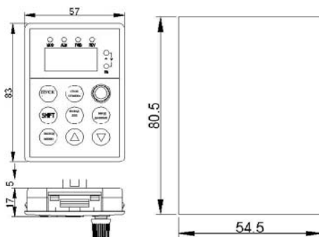
Рис. 2-5 Наружные размеры клавиатуры и ее соединительной коробки
